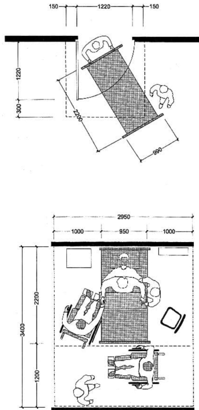
Рисунок Б.13 - Зоны обслуживания и зоны проезда в палатах для лежачих больных
