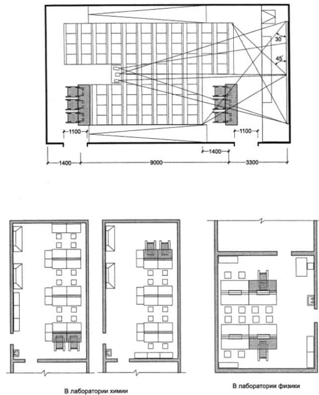
Рисунок Б.4 - Примеры расстановки оборудования в аудитории и лабораториях химии и физики
