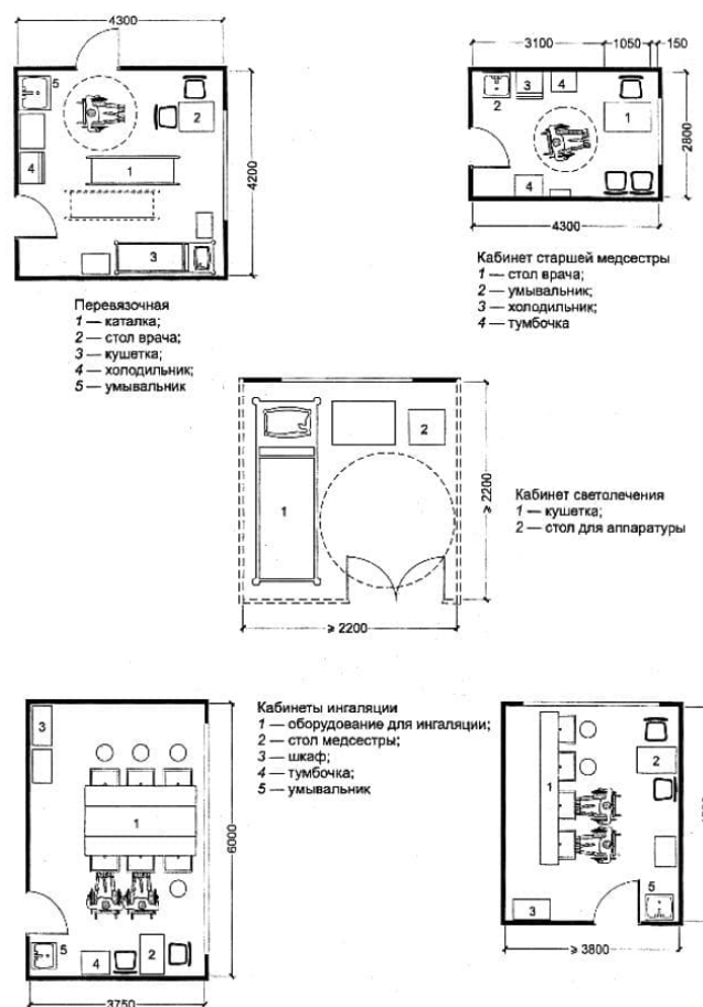
Рисунок Б.9 - Примеры расстановки оборудования в помещениях поликлиник и амбулаторий
