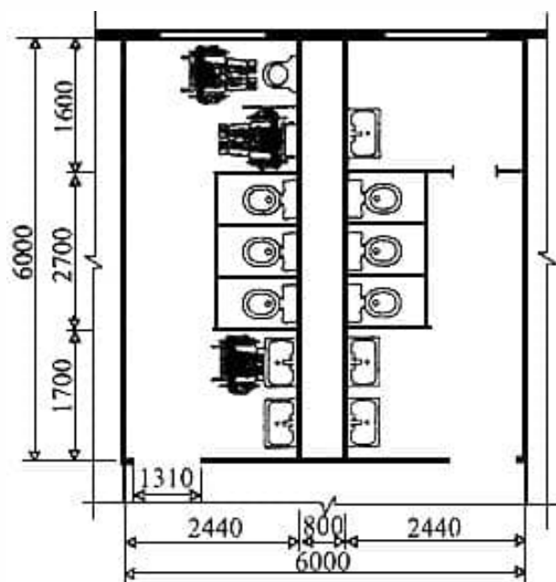
Цеховая уборная с кабиной для инвалидов
