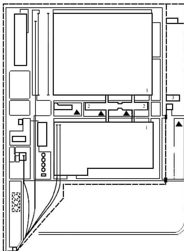
Рисунок В.1 - Рассредоточенное размещение личного транспорта инвалидов
