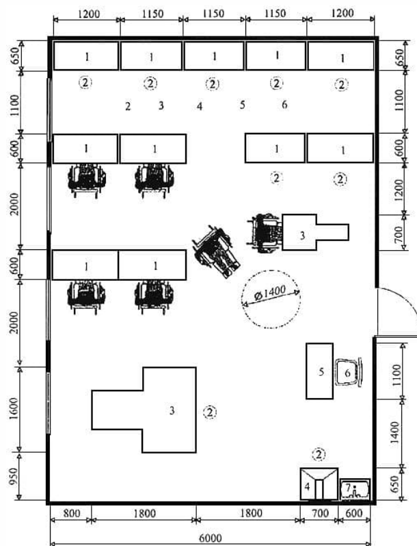
Рисунок В.11 - Пример планировки помещения. Картонажный участок, приспособленный для труда инвалидов в тарном цехе завода
