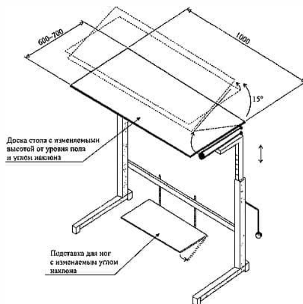
Рисунок В.12 - Трансформируемый рабочий стол для инвалида
