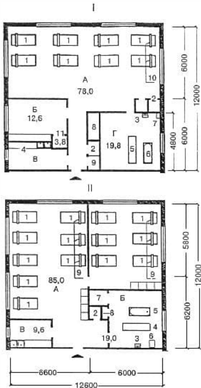
I - план. схема жилых комнат жилой ячейки типа 1в для лежащих детей с сохранным интеллектом
